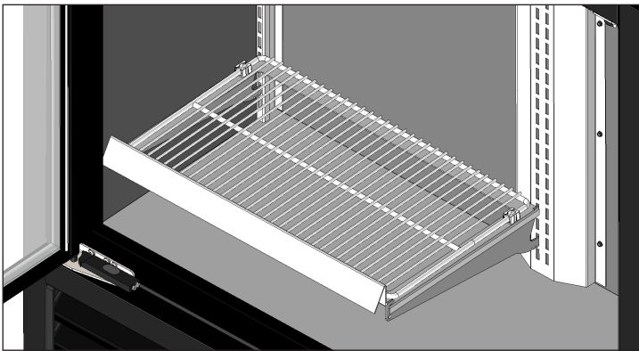
Fig. 17. Estante de rejilla en voladizo montado.
