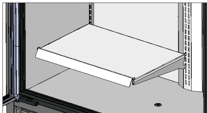
Fig. 10. Estante sólido en voladizo montado.
