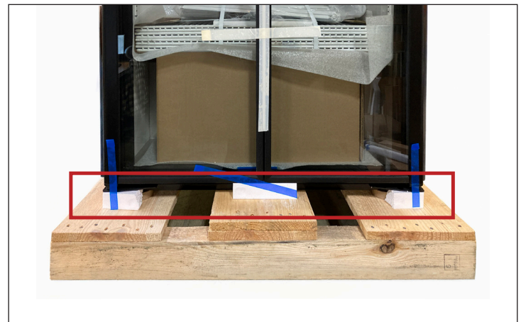
Fig. 1. Bloques de transporte de la puerta.
