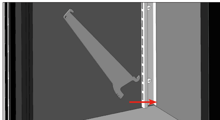
Fig. 6. Enganche la ménsula en las ranuras del perfil para estantes.
