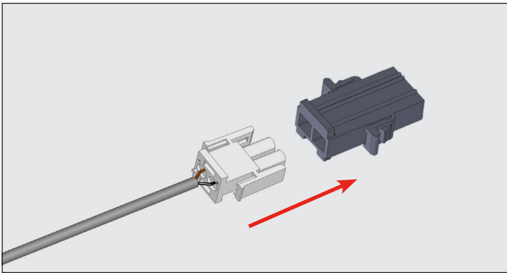
Fig. 2. Conector molex del letrero y receptáculo del área del letrero.
