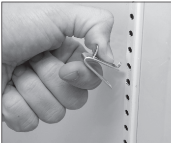
Fig. 1. Instalación de la pestaña superior del elemento de fijación del estante.
