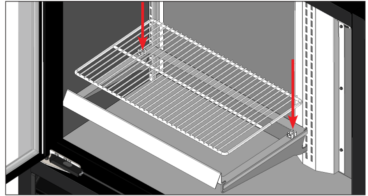
Fig. 16. Encaje el estante de rejilla en los elementos de fijación.
