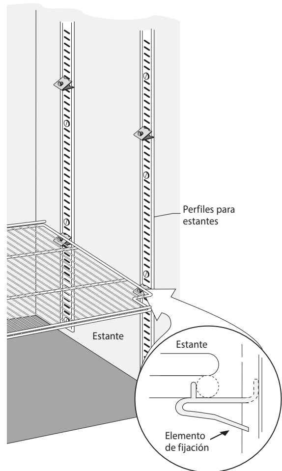
Fig. 3. Es posible que tenga que presionar o girar la parte inferior del elemento de fijación para instalarlo.
