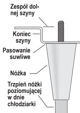
Rys. 4. Wkręcić nóżki poziomujące.
