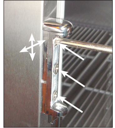
Fig. 4. Ubicación de los tornillos de las bisagras de la puerta. Mueva la bisagra según sea necesario.
