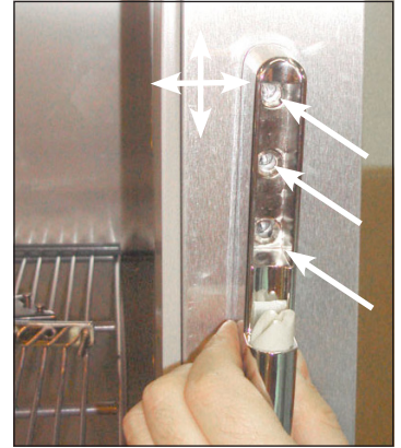
Fig. 2. Ubicación de los tornillos de bisagra del gabinete. Mueva la bisagra según sea necesario.
