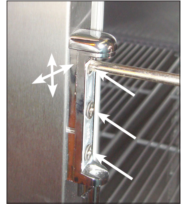
Abb. 4. Orte der Scharnierschrauben der Tür. Bewegen Sie das Scharnier, falls nötig.
