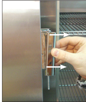
Abb. 3. Ziehen Sie die Scharnierabdeckung vom Türscharnier.
