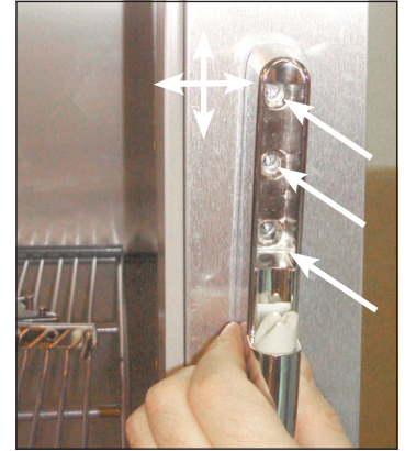
Abb. 2. Orte der Scharnierschrauben des Schrankes. Bewegen Sie das Scharnier, falls nötig.
