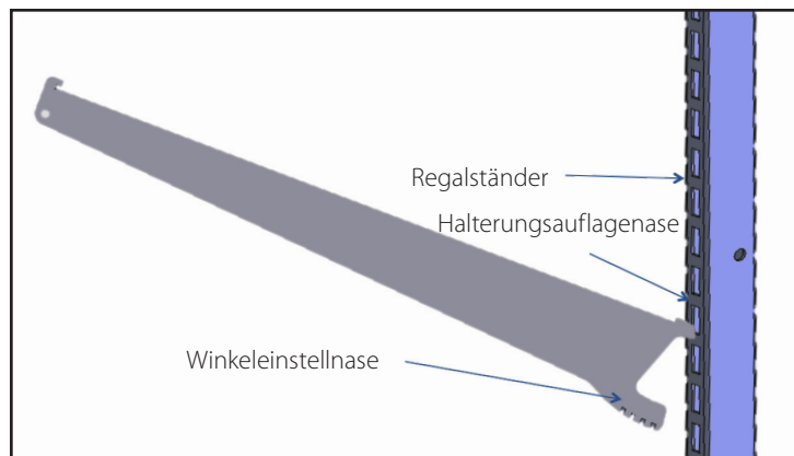
Abb. 1. Regalbretthalterungen einbauen.
