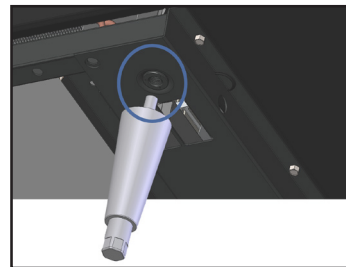
Abb. 3. Suchen Sie die Gewindebohrung in der Schiene.
