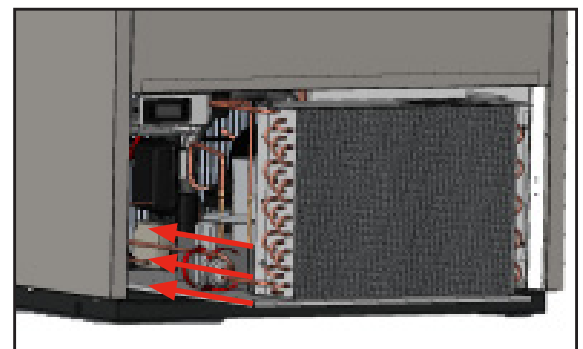
Abb. 7. Kondensatoreinheit austauschen.
