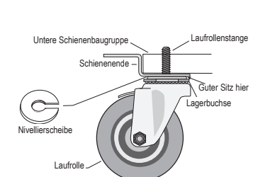
Abb. 7. Unterlegscheibe(n) installieren.
