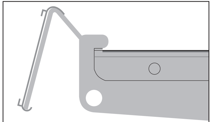
Abb. 3. Korrekter Einbau des Preisstreifens.
