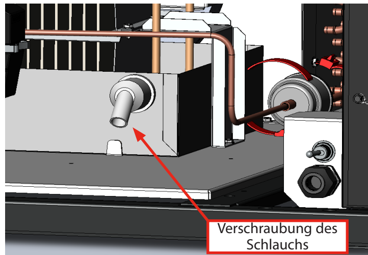
Abb. 1. Rückseite des Schrankes mit entferntem Drahtgitter.
