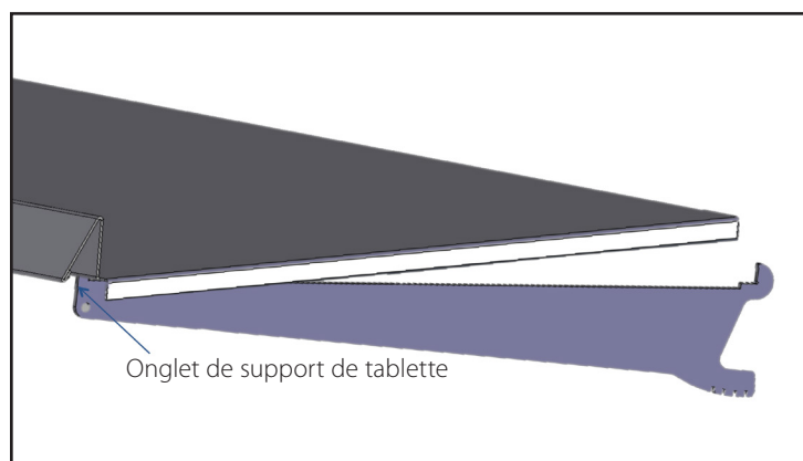
Fig. 2. Pose des clayettes.
