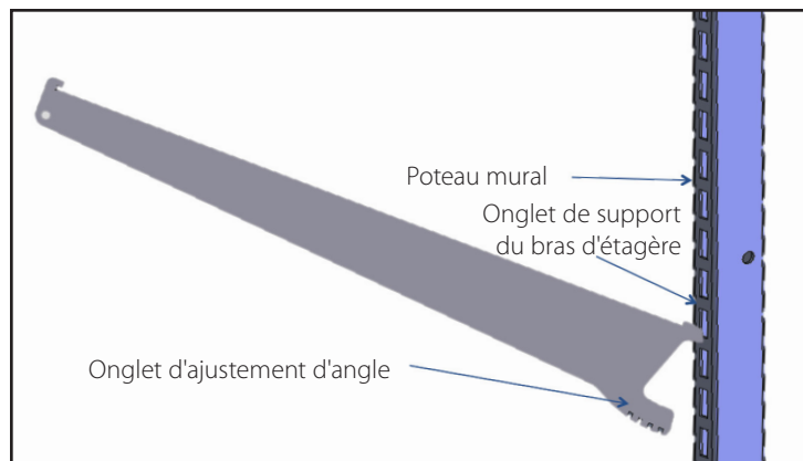
Fig. 1. Pose des consoles de clayette.
