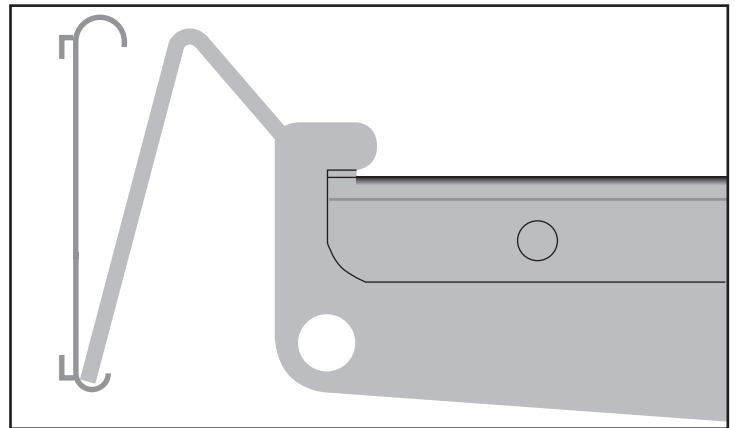
Fig. 2. Positionnement correct de la languette de clayette pendant la pose.
