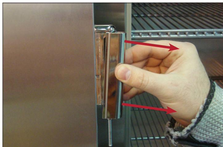
Rys. 3. Odciągnąć pokrywę zawiasów od zawiasów drzwi.
