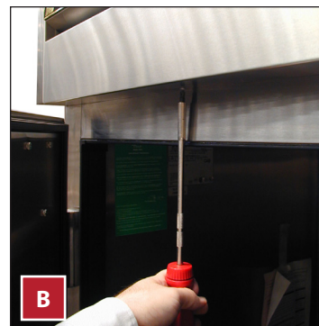
Rys. 2. Jeśli jest dostęp do węzownicy skraplacza, oczyścić ją. Nigdy nie należy czyścić szczotką węzownicy w poprzek uźebrowania.
