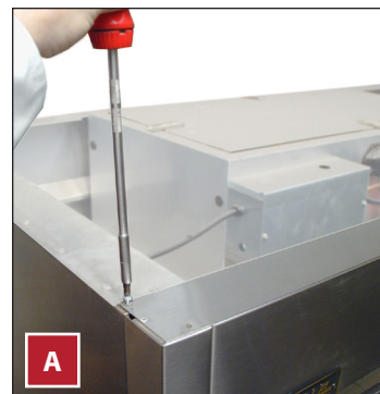
Abb. 3. Regenabweiser entfernen.
