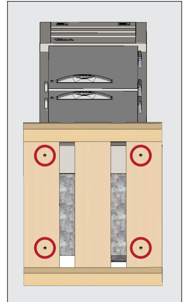
Abb. 2. Position der Transportsicherungen.
