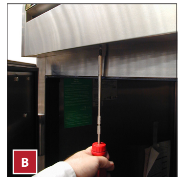
Abb. 2. Falls zugänglich, reinigen Sie die Kondensatorrohrschlange. Verwenden Sie die Bürste nicht an den Lamellen der Rohrschlange.
