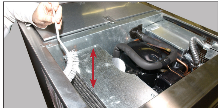
Abb. 2. Falls zugänglich, reinigen Sie die Kondensatorrohrschlange. Verwenden Sie die Bürste nicht an den Lamellen der Rohrschlange.
