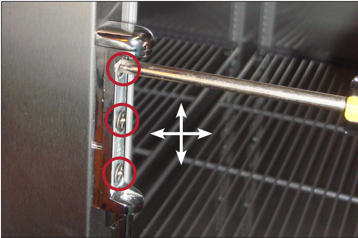
Abb. 4. Orte der Scharnierschrauben der Tür. Passen Sie das Scharnier nach oben, nach unten oder zur Seite hin an.
