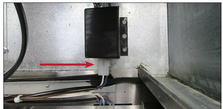
Abb. 4. Trennen Sie die elektronische Temperaturregelung.
