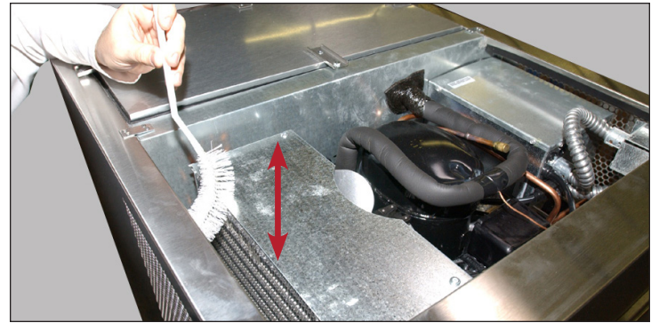
الشكل 2. إذا كان من الممكن الوصول إليها، نظف ملف المكثف. لا تستخدم الفرشاة أبدًا عبر زعانف السلك.
