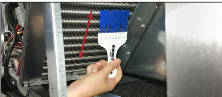
Fig. 3. Nunca pase el cepillo en perpendicular a las aletas del serpentín.
