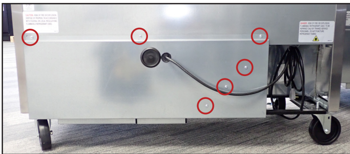
Рис. 2. Удалите винты из задней крышки (TFP/TSSU/TUC/TWT).
