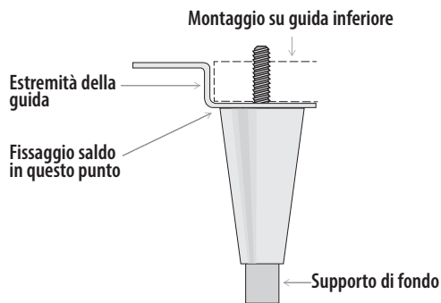
Fig. 4. Schema piedino di livellamento.
