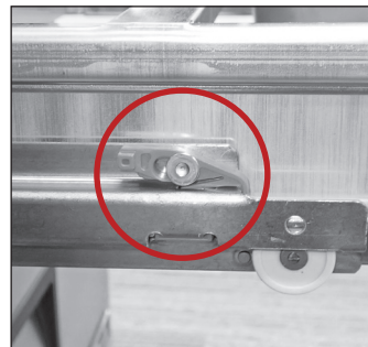
Fig. 5. Posizione del fermo del cassetto. Il fermo è inserito.
