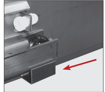
Fig. 2. Fermi delle rotelle in posizione abbassata.
