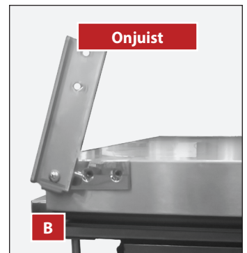
Afb. 8. Op de afbeeldingen is de voorkant van de deur naar boven gericht.
