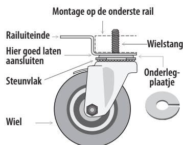
Afb. 7. Tekening wiel.
