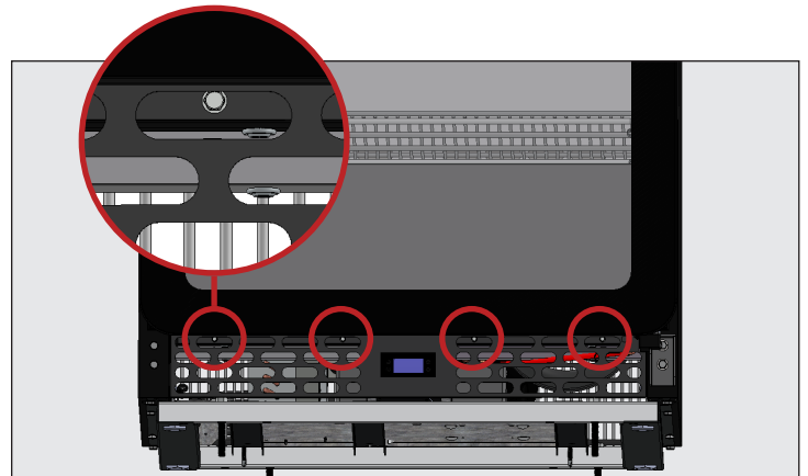
Fig. 3. Retire los pernos de la rejilla delantera para acceder a los pernos de transporte.
