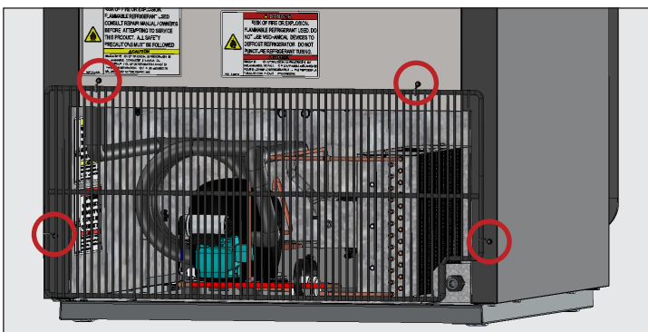
Рис. 2. Местонахождение винтов крепления задней решетки на модели CVM-20/24/27
