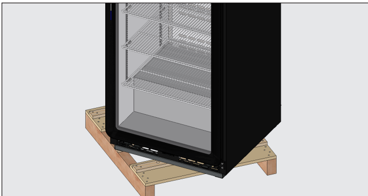
Abb. 4. Drehen Sie das Gerät auf der Kufe. Verwenden Sie beim Hochheben des Geräts keine Arbeitsplatten, Türen/Schubladen oder Gitter als Hebepunkte.
