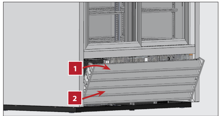
Fig. 8. Porte coulissante verticale : Incline le haut de la grille vers l'avant, puis soulevez-la.
