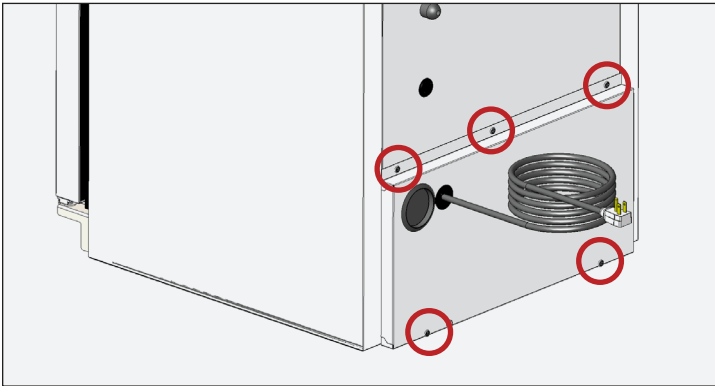
Fig. 3. Emplacements des vis du cache arrière.
