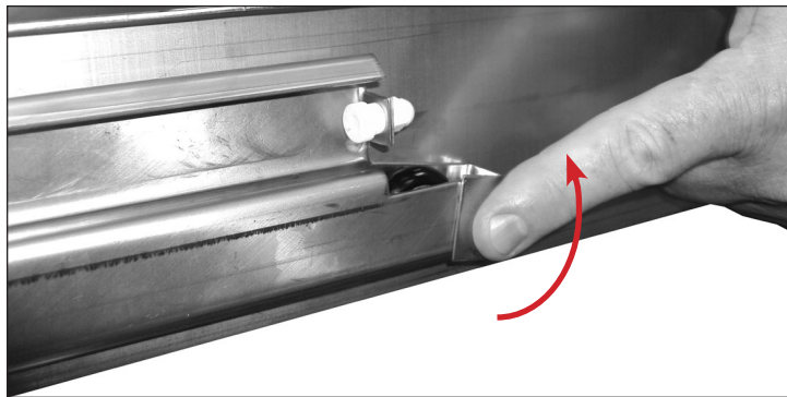
Rys. 3. Obrócić zatrzask rolki w górę.
