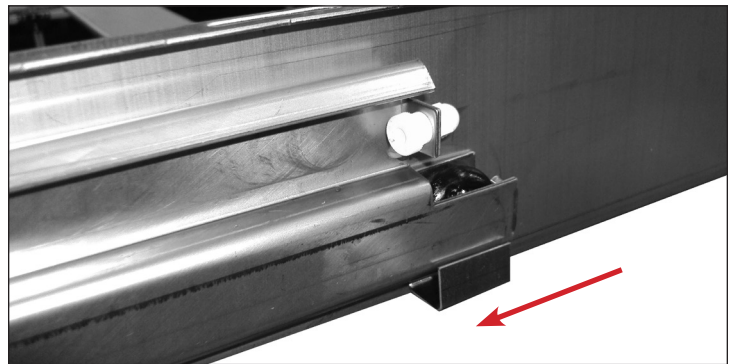
Fig. 2. Clip de rouleau en position basse.
