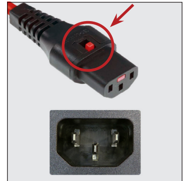
Şekil 2. Fiş çıkartmak için kırmızı butona basın.
