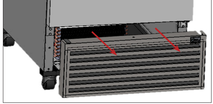
Şekil 2. Dikkatlice kafesi sökün.
