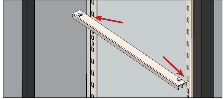
Şekil 1. Yuvaları kerkiklerle hizalayın.
