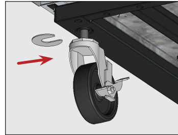
Şekil 9. Tekerlek ayar sacını/saclarını yerleştirin ve tekerlek sapını sıkıttığınızdan emin olun.
