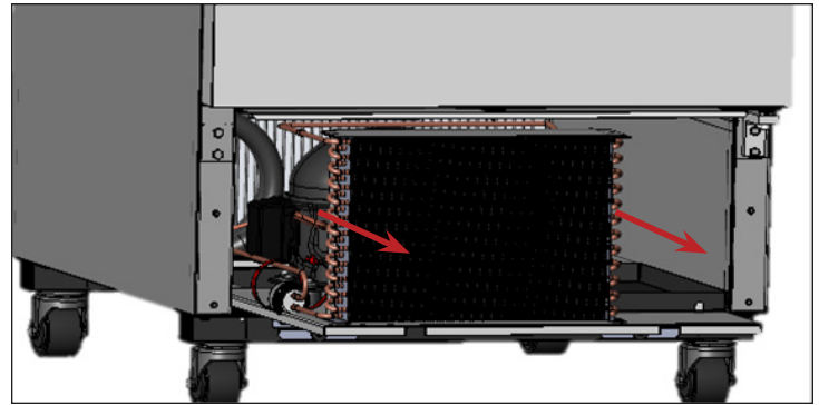
Şekil 6. Kondenser ünitesini dikkatlice kaydırarak çıkartın.
