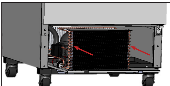
Fig. 7. Riportare con attenzione l'unità di condensazione in posizione e reinserire i bulloni.
