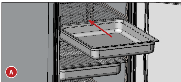
Fig. 4. Scorrimento del ripiano/vaschetta installato.
