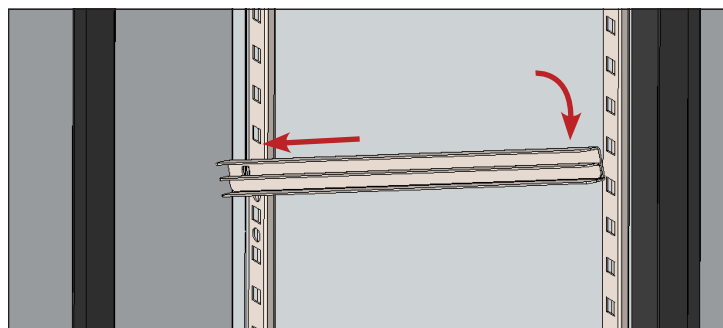
Fig. 2. Posizionare lo scorrimento del ripiano/vaschetta.
