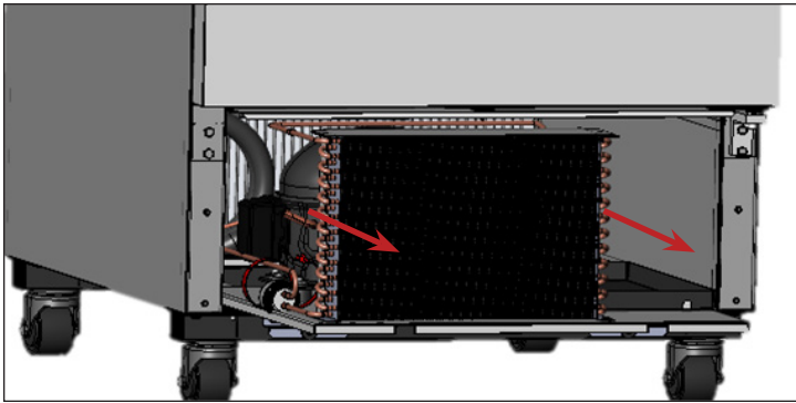
الشكل ٦. حرك وحدة التكثيف إلى الخارج بحرص.
