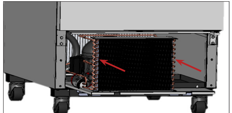
الشكل ٧. أعد تحريك وحدة التكثيف بحرص إلى موضعها، وأعد تركيب المسامير.
