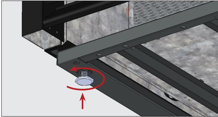
الشكل ٣. أدبر برغي ضبط الاستواء عكس اتجاه عقارب الساعة لرفع الجهاز.
