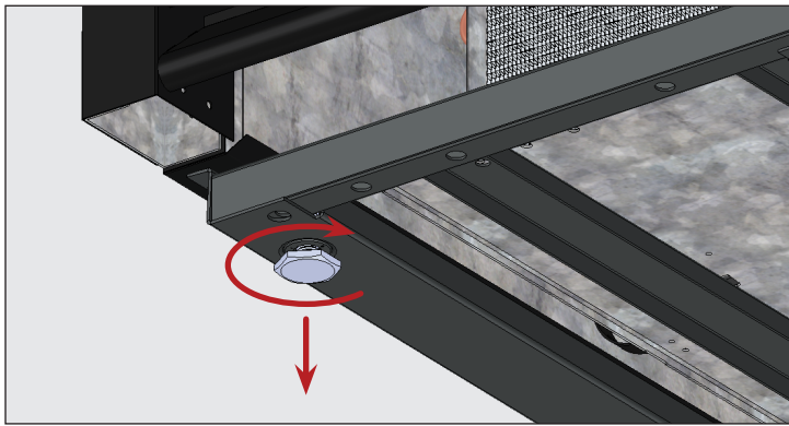
الشكل ٢. أدبر برغي ضبط الاستواء في اتجاه عقارب الساعة لخفض الجهاز.
