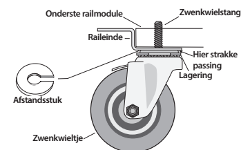
Afb. 7. Installeer de (het) onderlegplaatje(s).
