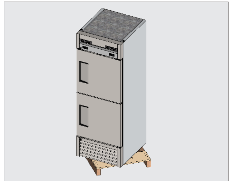
Fig. 4. Al elevar la unidad, no use encimeras, puertas, cajones ni rejillas como punto de elevación.
