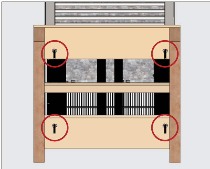
Fig. 3. Ubicaciones de los pernos de transporte.
