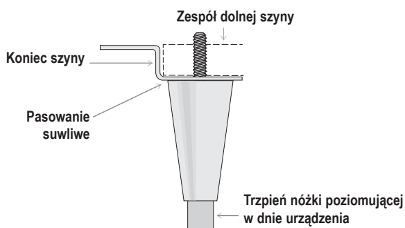
Rys. 4. Rozmieszczenie nóżek poziomujących.
