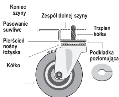
Rys. 7. Rozmieszczenie kółek.
