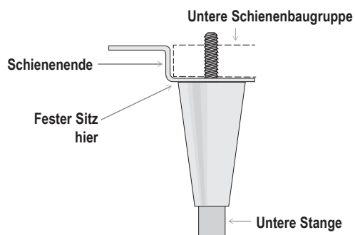
Abb. 4. Nivellierbein-Diagramm.
