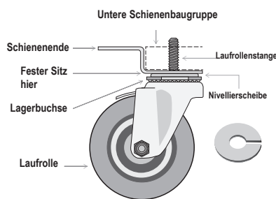
Abb. 7. Rollendiagramm.
