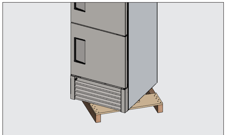
Fig. 4. Al elevar la unidad, no use encimeras, puertas, cajones ni rejillas como punto de elevación.
