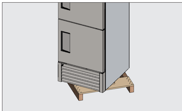
Figura 4. Quando si solleva l'elettrodomestico, non utilizzare banconi di lavoro, sportelli/cassetti o griglie come punti di sollevamento.
