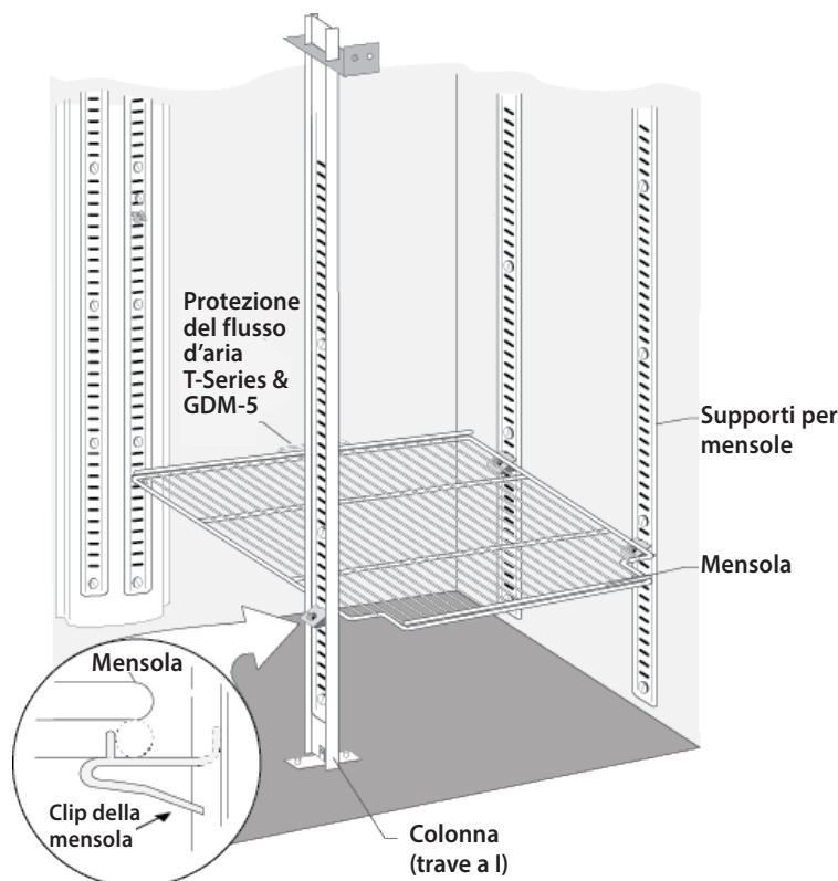
Figura 3. Potrebbe essere necessario stringere o girare leggermente la clip della mensola per facilitarne l'installazione
