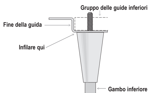
Fig. 4. Diagramma della gamba di livellamento
