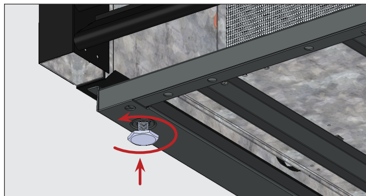
Figura 3. Girare le viti di livellamento in senso antiorario per sollevare l'elettrodomestico.
