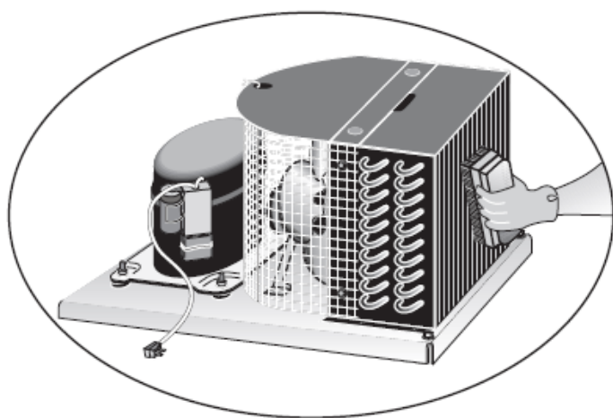
Figura 2. Con una spazzola a setole dure, pulire con cautela lo sporco accumulato dalle alette frontali della bobina del condensatore.
