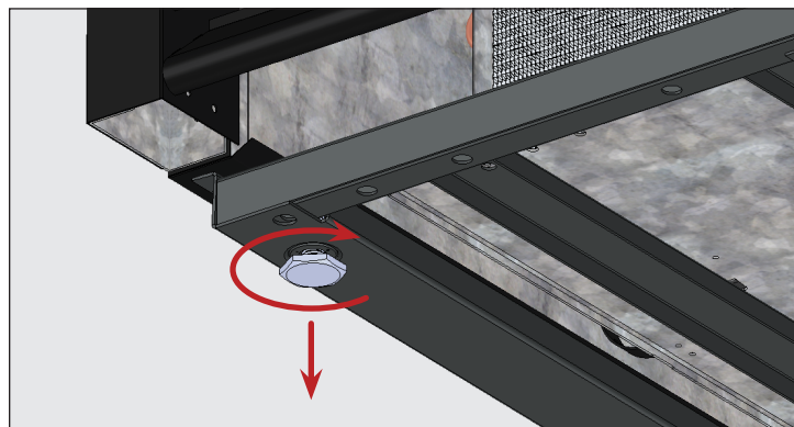
Figura 2. Girare le viti di livellamento in senso orario per abbassare l'elettrodomestico.
