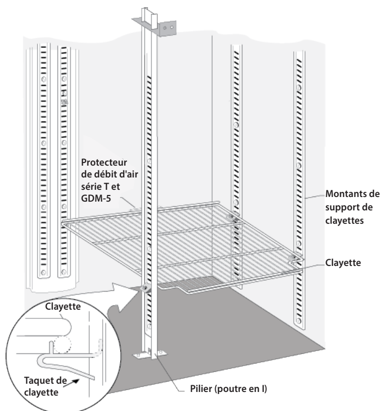
Figure 3. Vous devrez peut-être pincer ou tordre légèrement le bas du taquet de clayette pour la pose.
