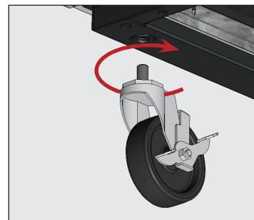
Fig. 8. Atarraxe os rodízios nos furos rosçados.
