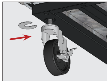
Fig. 9. Inserire la/le zeppa/e della rotella orientabile. Assicurarsi di stringere bene il perno della rotella orientabile.
