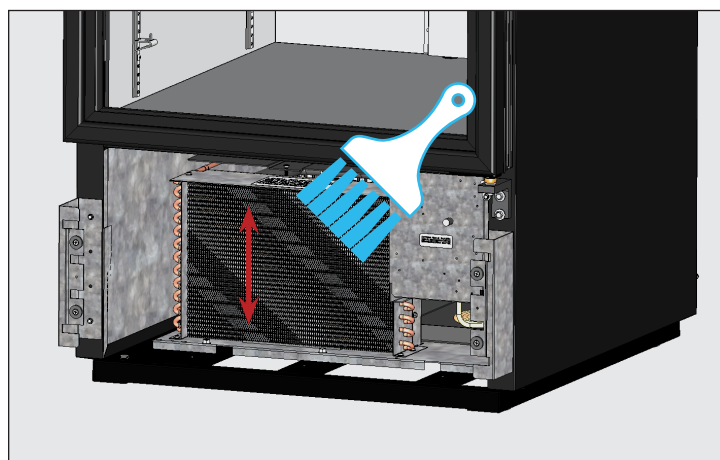
Fig. 4. Non spazzolare mai sulle alette della bobina.
