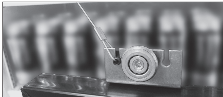
Fig. 9. Assicurarsi che il cavo dello sportello sia nello spazio del rullo più vicino alla puleggia.
