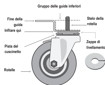
Fig. 7. Diagramma della rotella orientabile.
