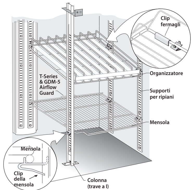
Fig. 5. I modelli GDM-5 includono una protezione per il flusso d'aria sulla parte posteriore degli scaffali per mantenere uno spazio d'aria sul retro dell'elettrodomestico.
