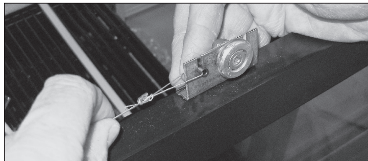
Fig. 7. Togliere il cavo dello sportello dalla staffa del rullo.
