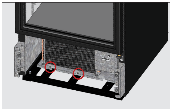
Abb. 6. Entfernen Sie die Schrauben an der Kondensatorbasis.
