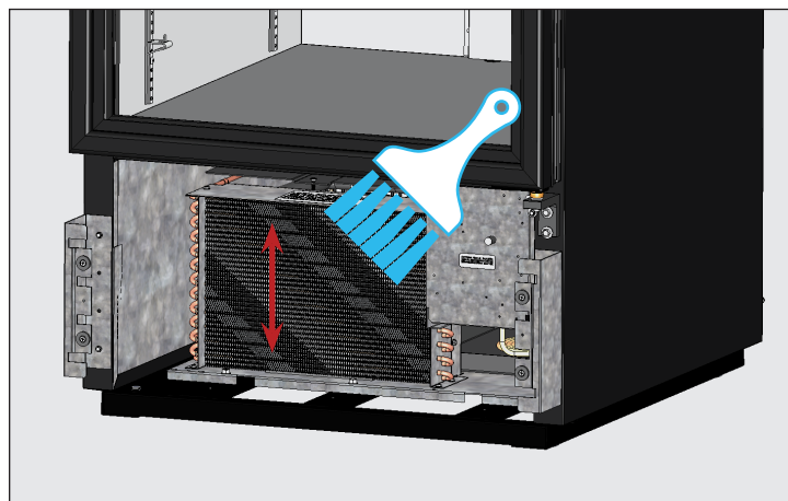
Abb. 4. Verwenden Sie die Bürste nie an den Lamellen der Rohrschlange.
