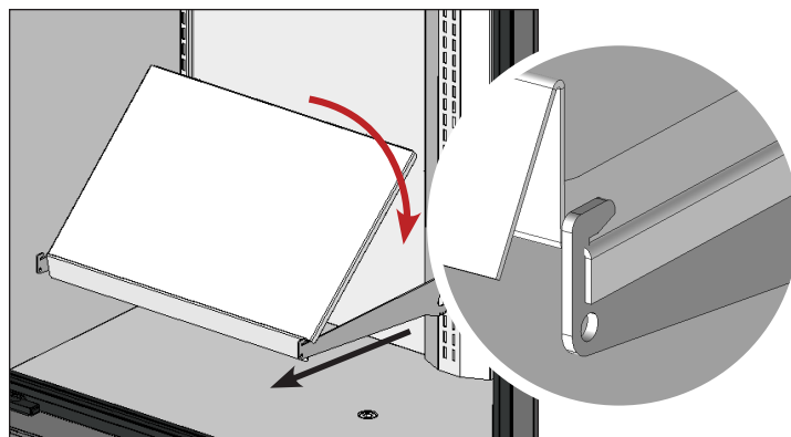
Abf. 5. Positionieren Sie das Regalbrett, während Sie die Rückseite des Regalbretts anheben. Achten Sie darauf, dass die Seiten des Regalbretts über der Halterung hängen.
