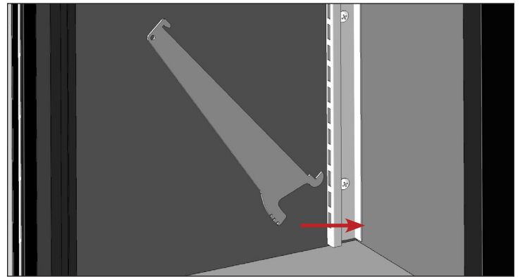
Abb. 2. Haken Sie den Bodenträger in die Regalständer ein.
