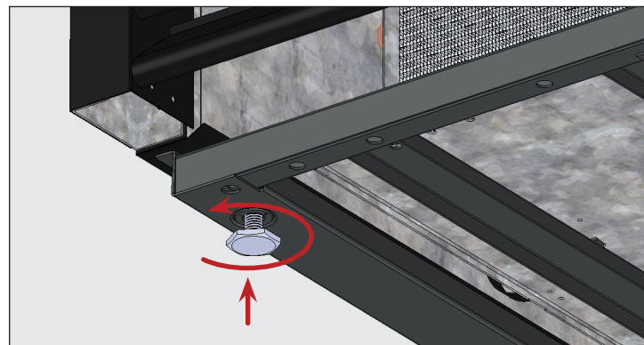
Abb. 3. Drehen Sie die Nivellierbeine gegen den Uhrzeigersinn, um das Gerät zu heben.
