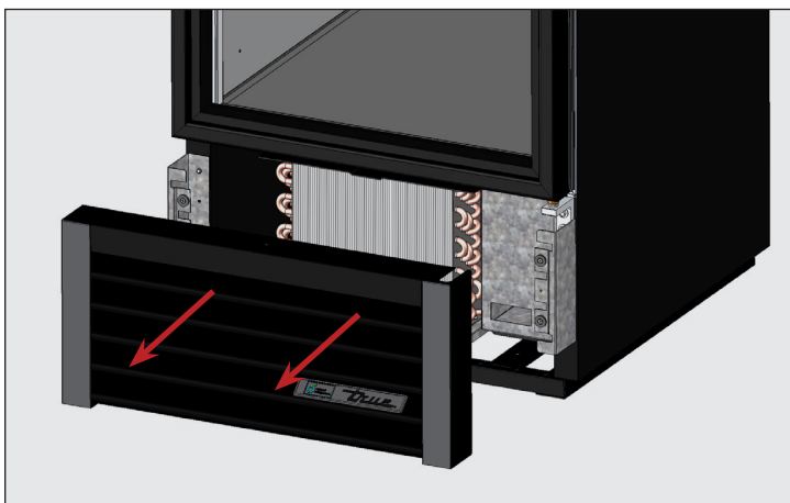
Abb. 3. Entfernen Sie vorsichtig das Gitter.
