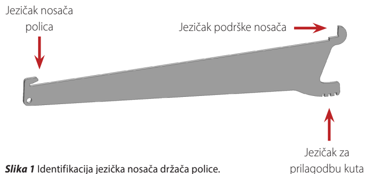
Slika 1 Identifikacija jezička nosača držača police.
