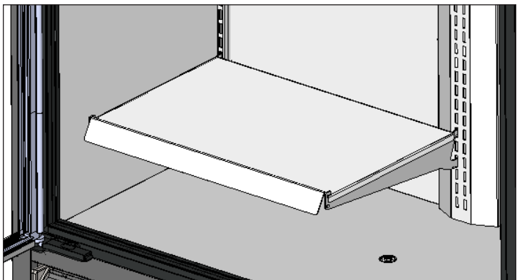
Slika 6 Ugrađena čvrsta konzolna polica.
