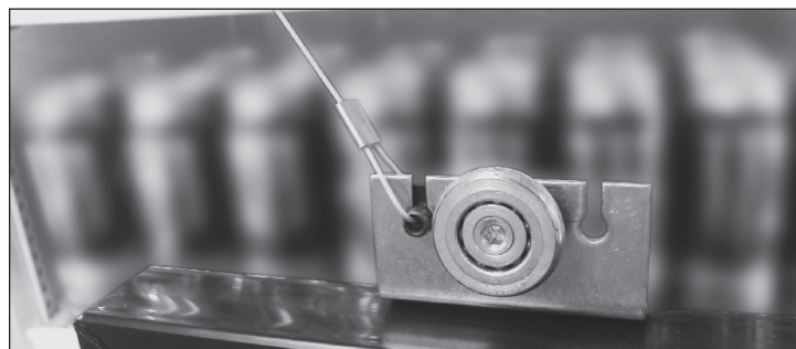
SI. 9. Provjerite je li kabl za vrata zakačen na kružni priključak najbliže mjestu povlačenja.
