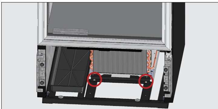
Abb. 5. Entfernen Sie die Schrauben an der Kondensatorbasis.
