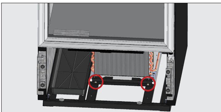
Figure 5. Déposez les vis du socle du condenseur.
