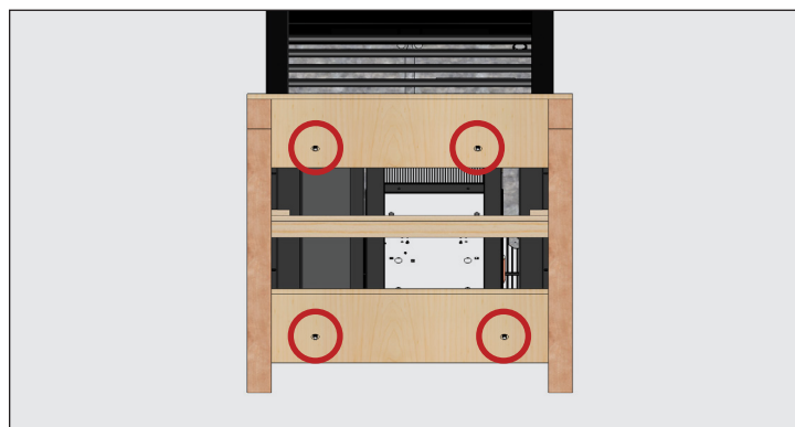
Figure 3. Emplacements des vis de transport.
