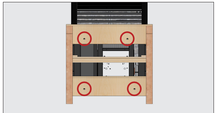
Afb. 3. Locaties van de transportbouten.
