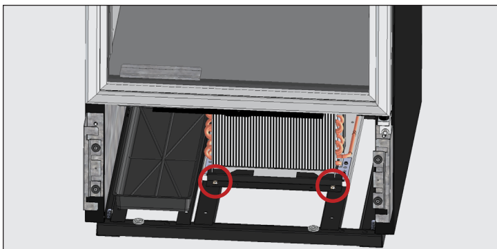
Afb. 5. Verwijder de bouten van de onderkant van de condensator.
