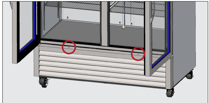
الشكل 1. مكان مسامير شبكة تهوية الباب المتأرجح.
