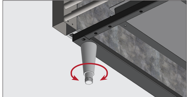
الشكل 6. لف الساق السفلي لاستواء الجهاز.
