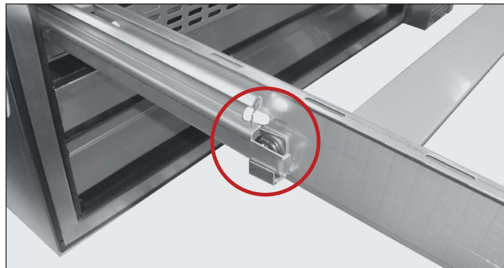
Fig. 1. Ubicación de las abrazaderas para rodillos.
