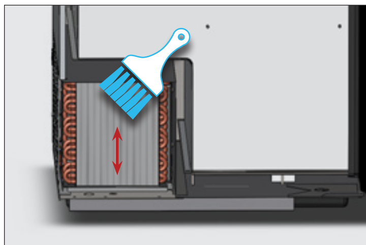
Fig. 4. Nunca cepille a través de las aletas del serpentín.
