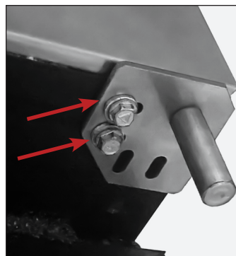
Fig. 9. Togliere il gruppo cartuccia del cardine dallo sportello.
