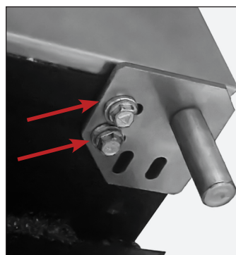
Fig. 9. N'oubliez pas les rondelles de la charnière.
