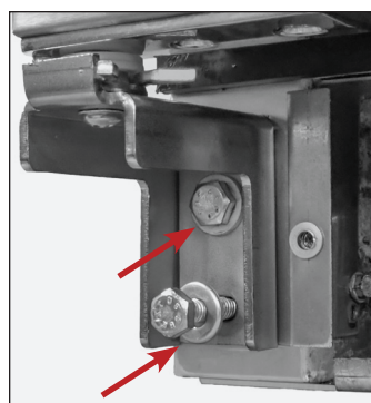
Fig. 11. N'oubliez pas les rondelles de la charnière.
