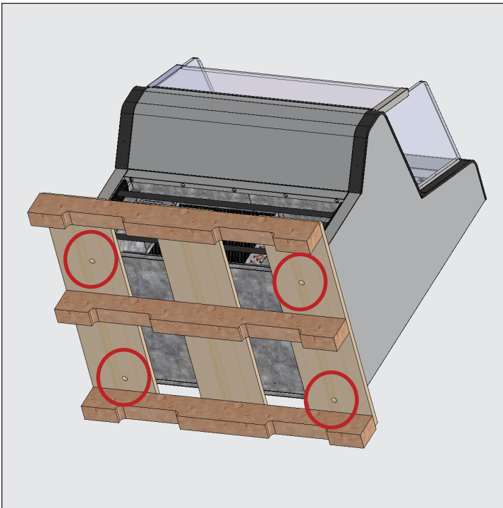
Abb. 2. Transportschrauben.
