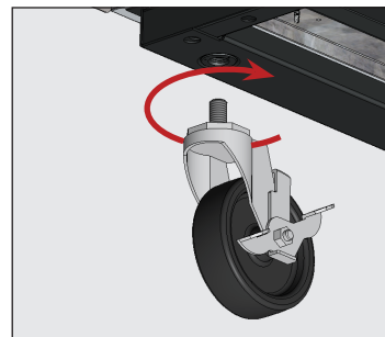
Abb. 5. Schrauben Sie die Lenkrollen in die Gewindebohrungen.
