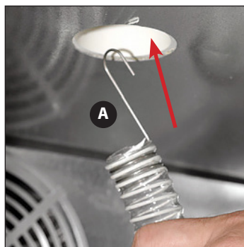
Fig. 8. Introduzca desde abajo la manguera de refrigeración en la torre de tiro (A) y engánchela en la parte superior del manguito aislante (B).
