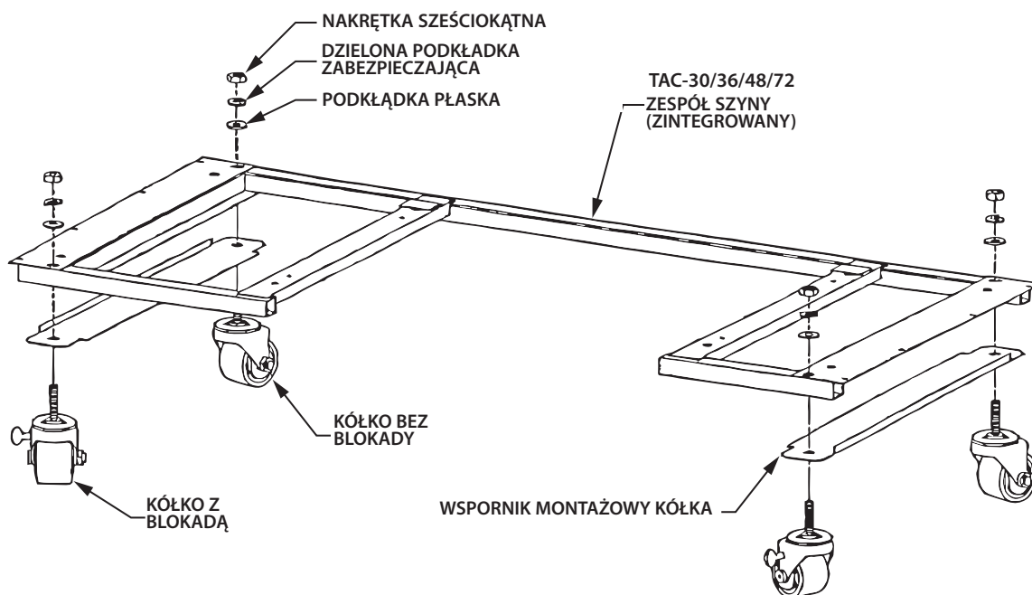
TAC-30/36/48/72 SCHEMAT MONTAZU ZETAWU KÓŁEK
