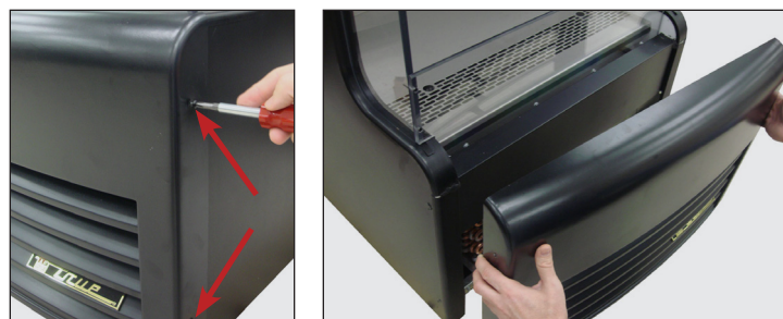
Rys. 2. TAC-14GS-HC-LD Demontaż kratki. Po wykręceniu śrub zdjąć w górę kratkę.
