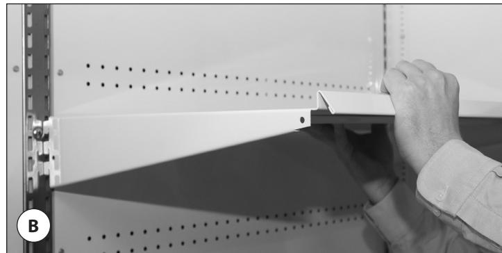
Rys. 2. Wczepić wsporniki półki w szyny półek.
