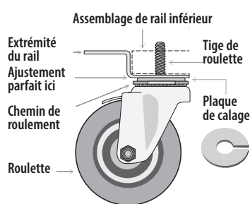
Fig. 7. Diagramme des roulettes.
