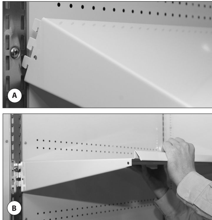
Fig. 2. Accrochez les supports d'étagère dans l'installation standard des étagères.
