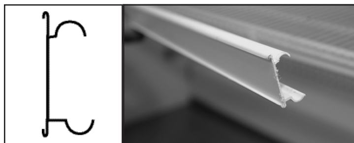
Fig. 2. Enclenchez le porte-étiquettes d'identification de produit sur l'étagère avec le côté le plus large en bas.
