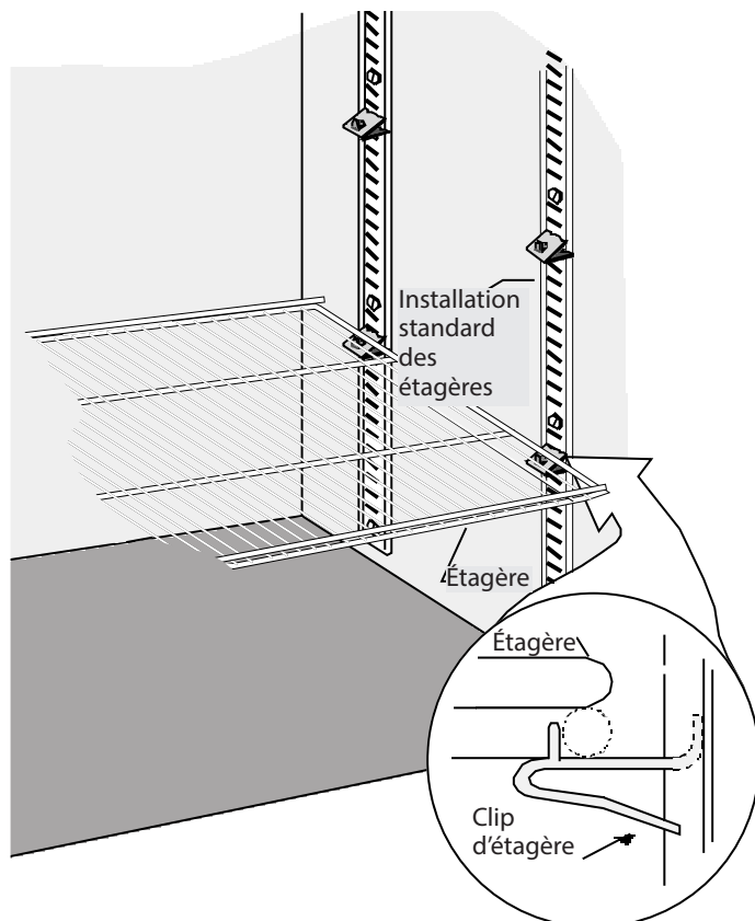
Fig. 8. Vous devrez peut-être serrer ou tourner le bas du clip d'étagère pour l'installer.
