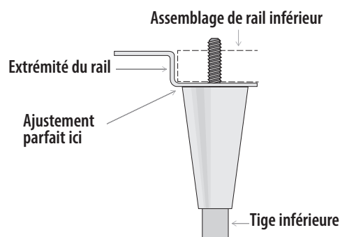
Fig. 4. Diagramme des pieds de mise à niveau.
