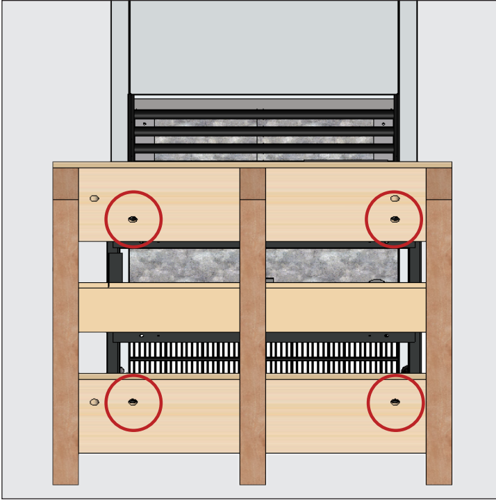
Şekil 2. Nakliye civatası konumları.
