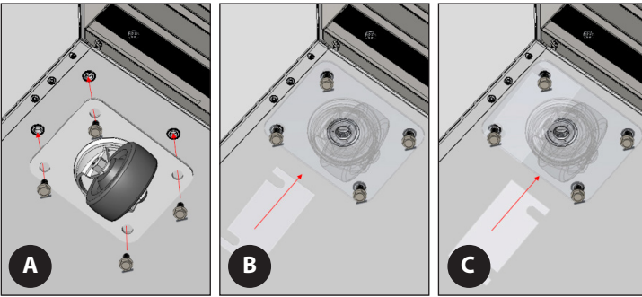
Şekil 7. Tekerlek takozlarını çiftler halinde takın.
