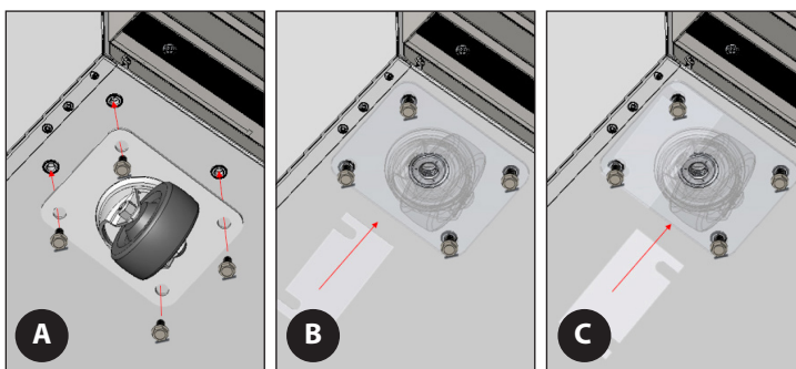
Fig. 7. Instale las cuñas de las ruedecillas en pares.
