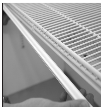
Fig. 3 Installare la striscia ID del prodotto.
