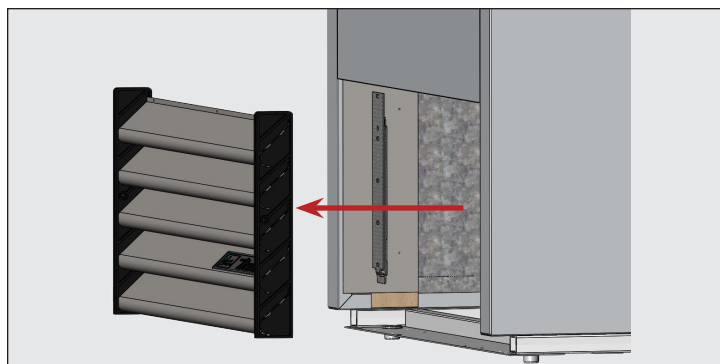
Abb. 2. Ziehen Sie, um das Lamellengitter zu entfernen.
