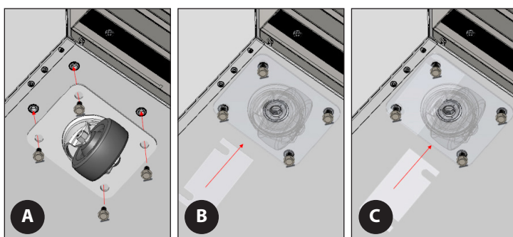
Fig. 7. Installez les cales de roulettes par paires.
