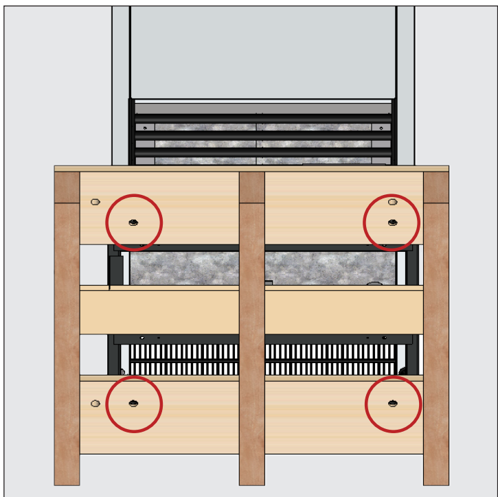
Fig. 2. Emplacements des vis de transport.
