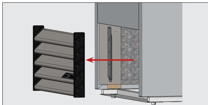
Afb. 2. Trek het rooster eruit.
